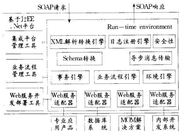
图 5 WSBI平台基本框架
