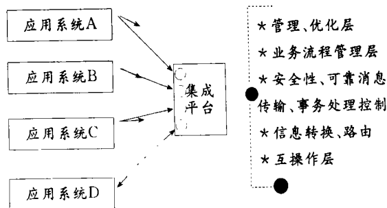
图 3 集成代理架构模式
