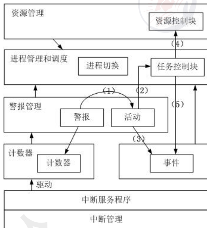
图 3-4 AUTOSAR 定义的操作系统结构
