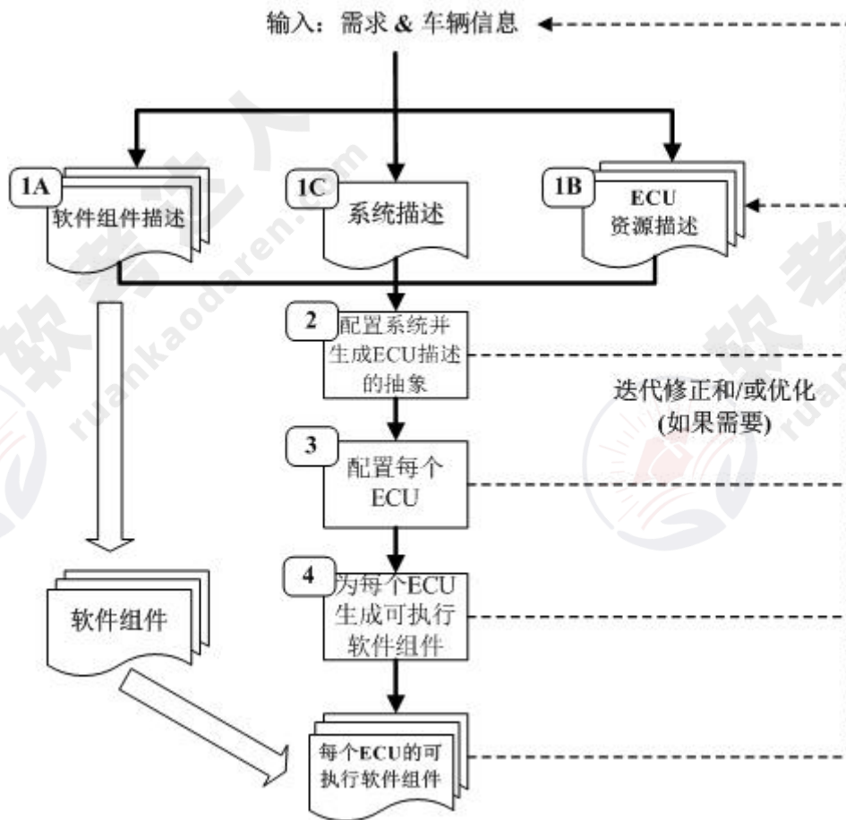
图 3-2 李工设计的流程
