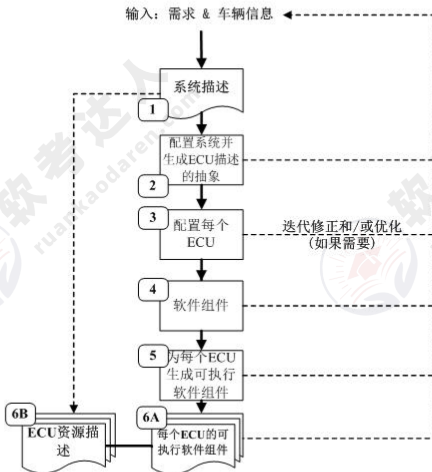
图 3-3 王工设计的流程
