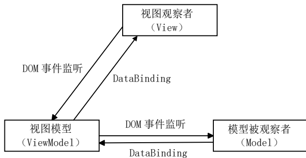
图 16.5 MVVM 流程设计模式
