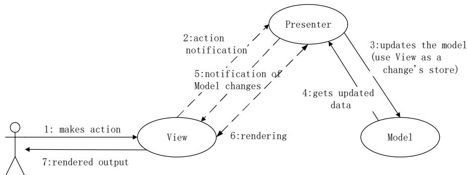
图 16.4 MVP 设计模式
