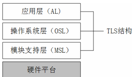
图 3.1 宇航嵌入式设备软件架构
