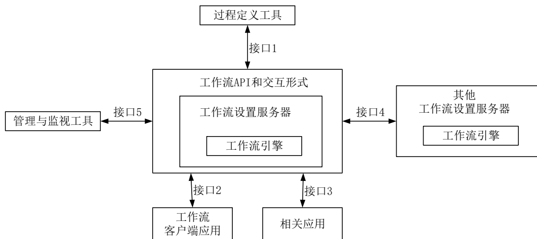
图 16.6 工作流参考模型
