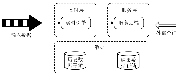
图 22.3 Kappa 架构
