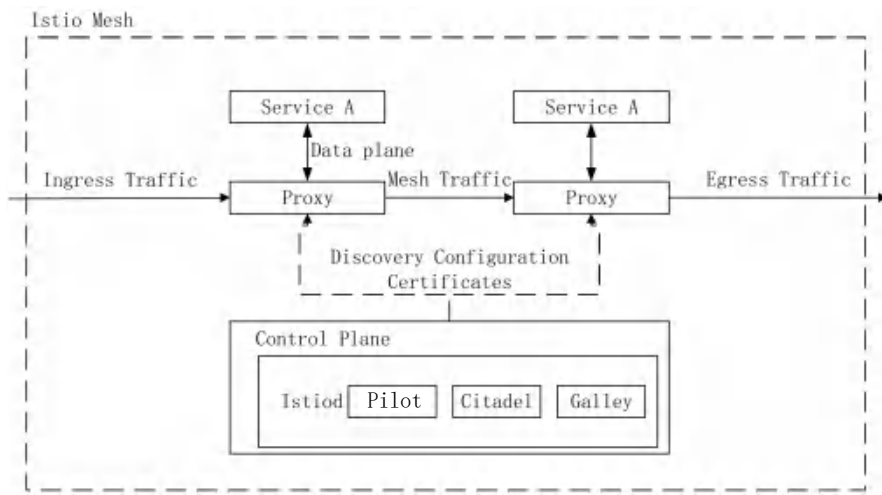
图 17.3 服务网络的典型架构
