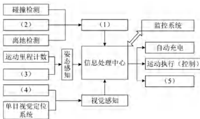
图 3.1 功能结构图
