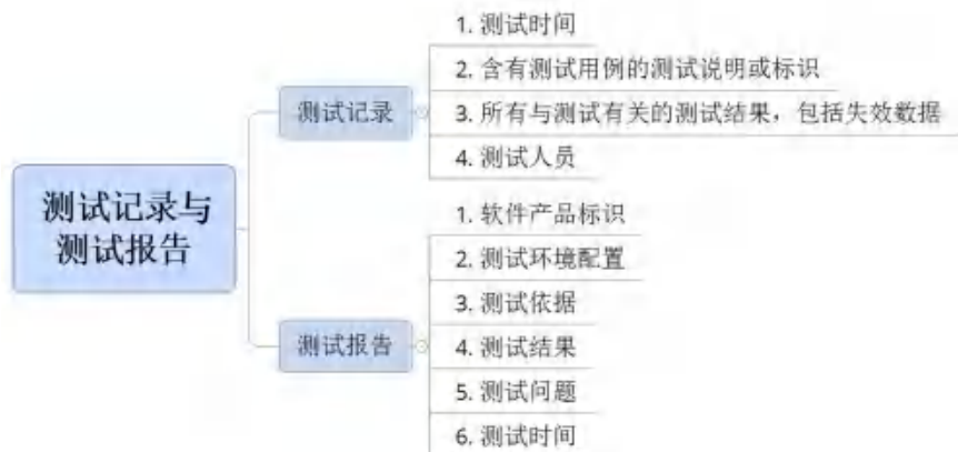
图 11.7 测试记录与测试报告的组成
