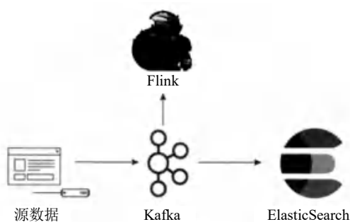
图 22.5 混合分析系统 Kappa 架构
