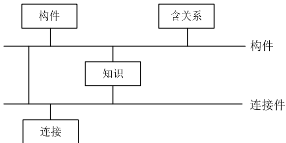
图 9.10 C2 风格
