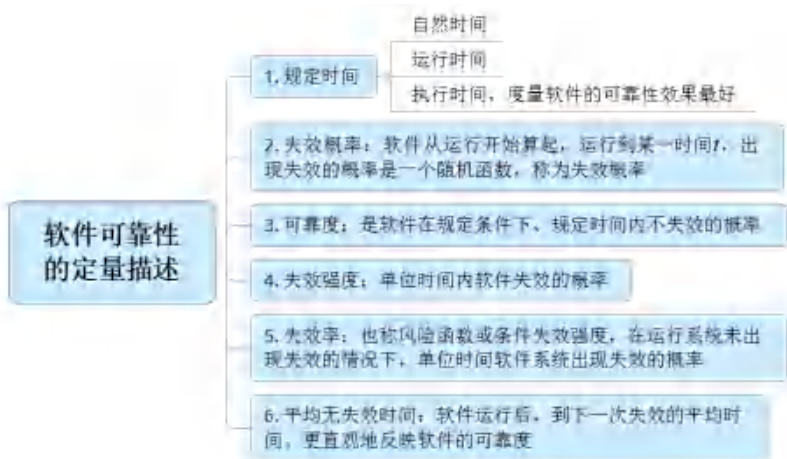
图 11.2 软件可靠性的定量描述
