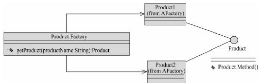
图 10-2 面向接口的简单工厂模式
