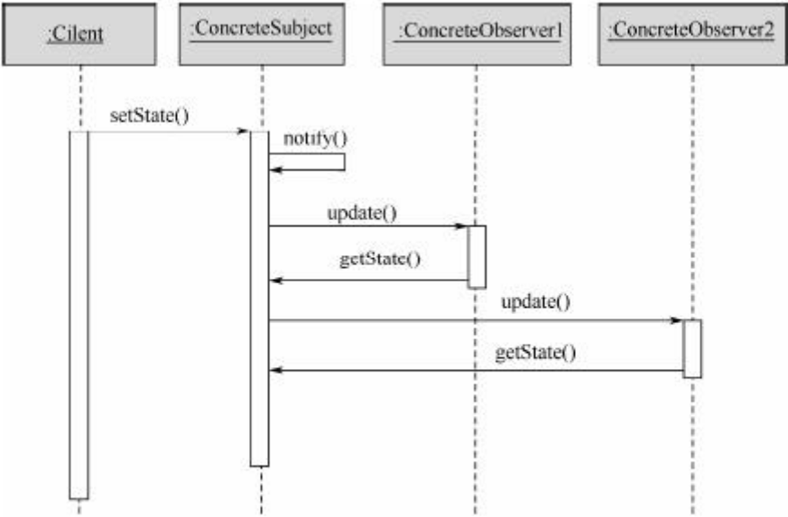
图 10-11 Observer 模式的工作方式
