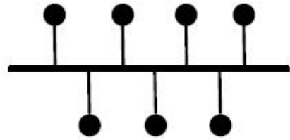
图 4-2 总线结构
