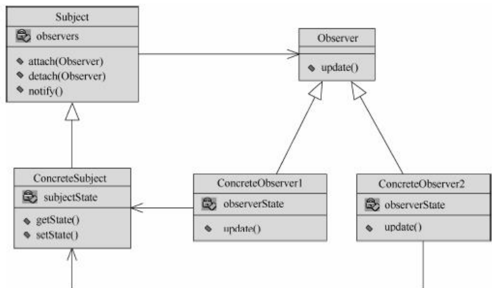
图 10-10 Observer 模式
