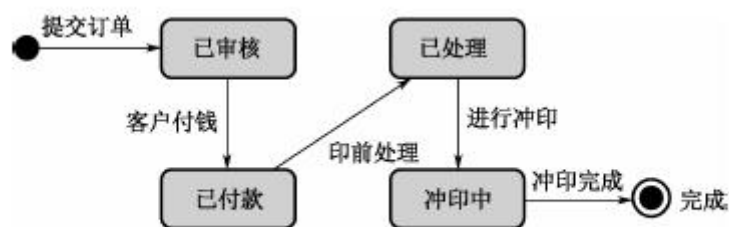
图 8-19 状态图示例
