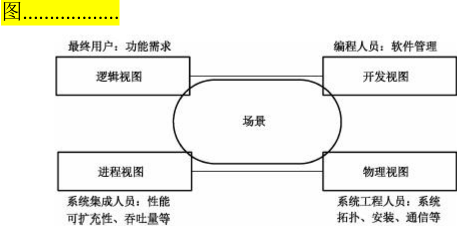
图 9-1 “4+1”视图模型
