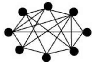
图 4-4 网状结构
