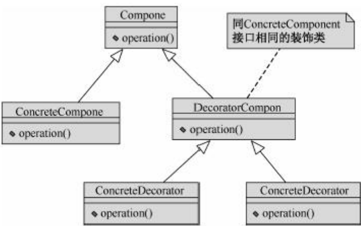
图 10-4 Decorator 模式
