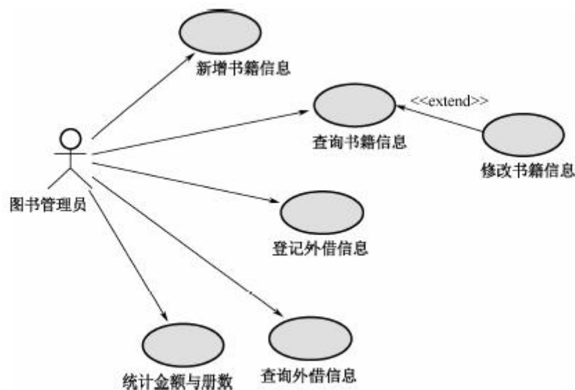
图 8-12 用例图示例
