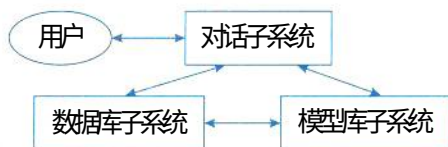
图3-12 DSS的两库结构
