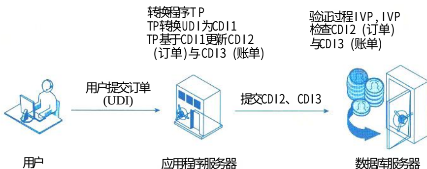
图18-7 CWM模型基本原理图
