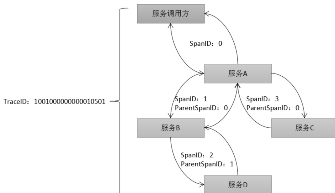
图1-15 通过TraceID串联起来的Trace
