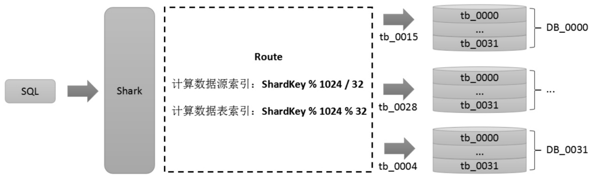
图5-7 Shark数据路由过程
