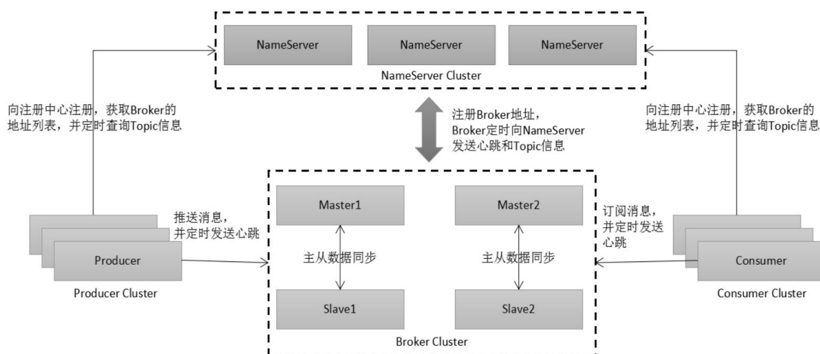
图2-9 RocketMQ的网络架构
