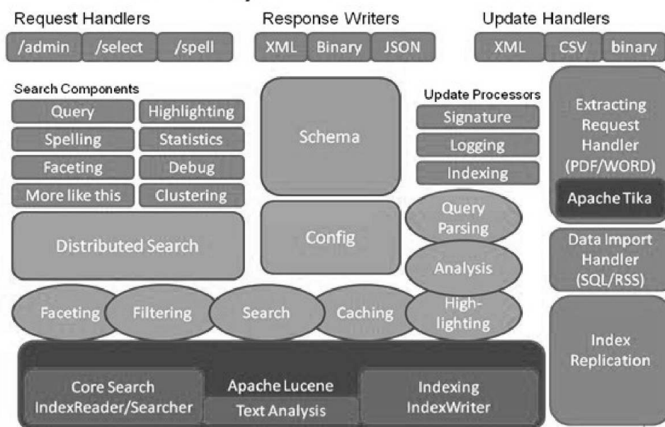
图5-9 Solr的整体架构
