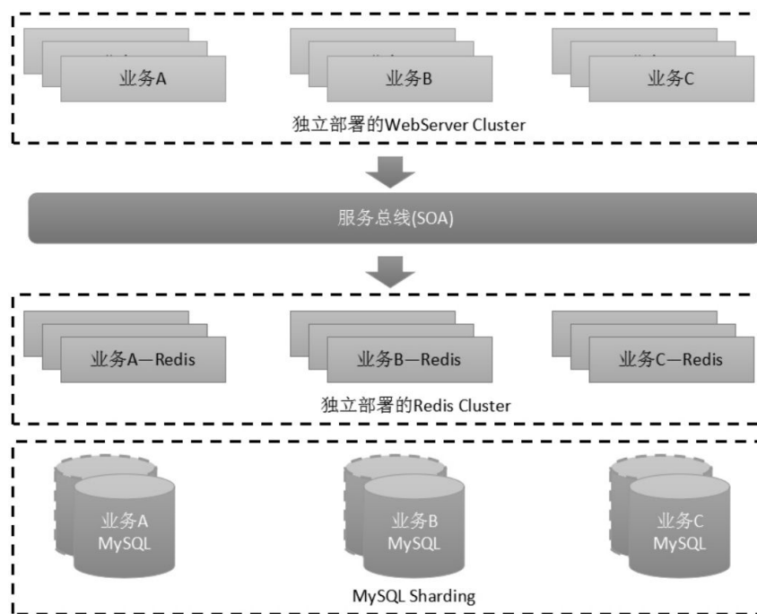
图1-6 服务化架构
