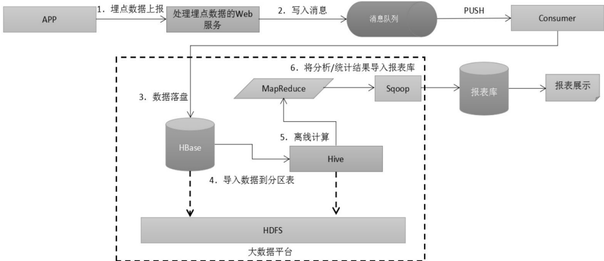
图2-10 前端埋点数据上报与离线分析流程
