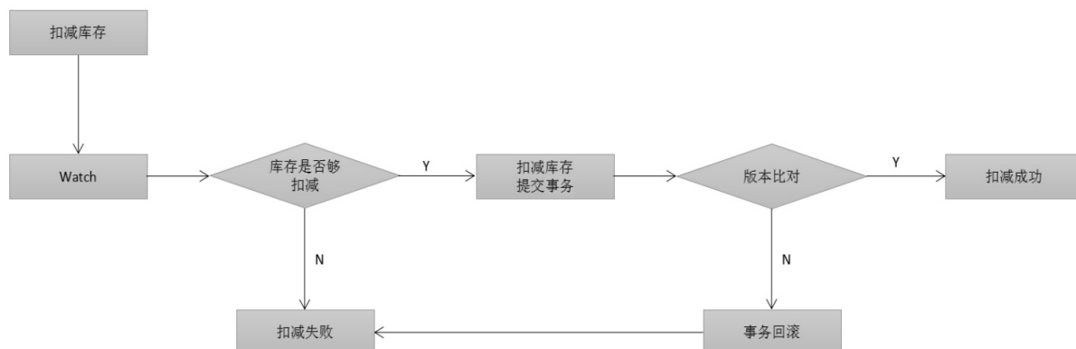
图4-13 采用乐观锁机制在Redis中扣减热卖商品库存
