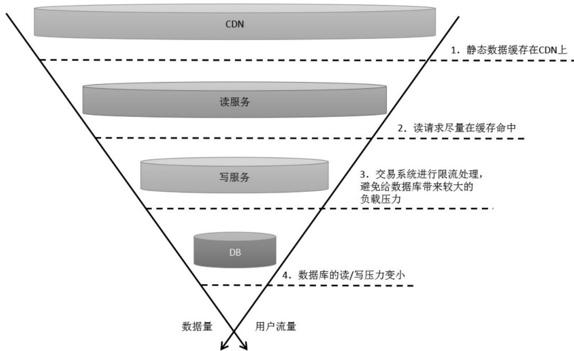
图2-2 漏斗模型
