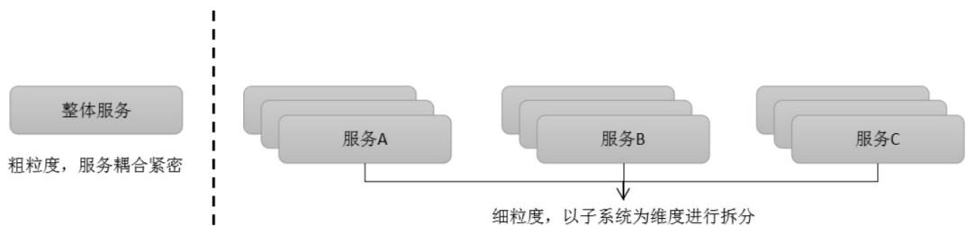
图1-7 微服务架构
