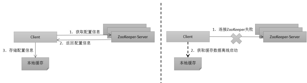
图3-9 客户端容灾
